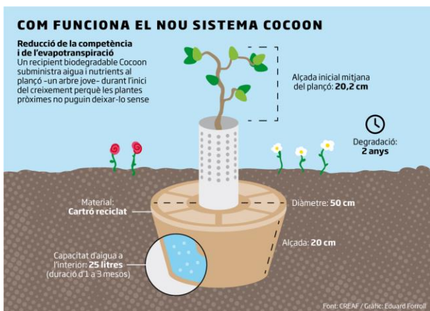
Figura 3. Esquema de funcionament del sistema Cocoon. (Font: CREA).
